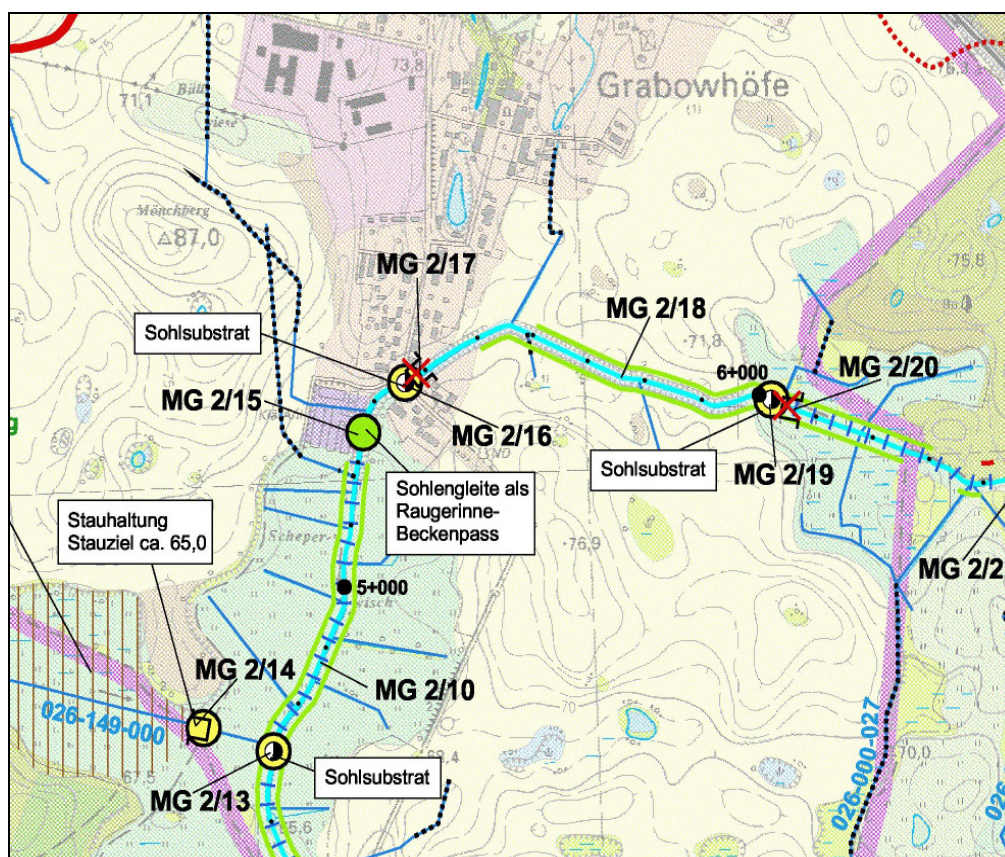
Ausschnitt Lageplan
