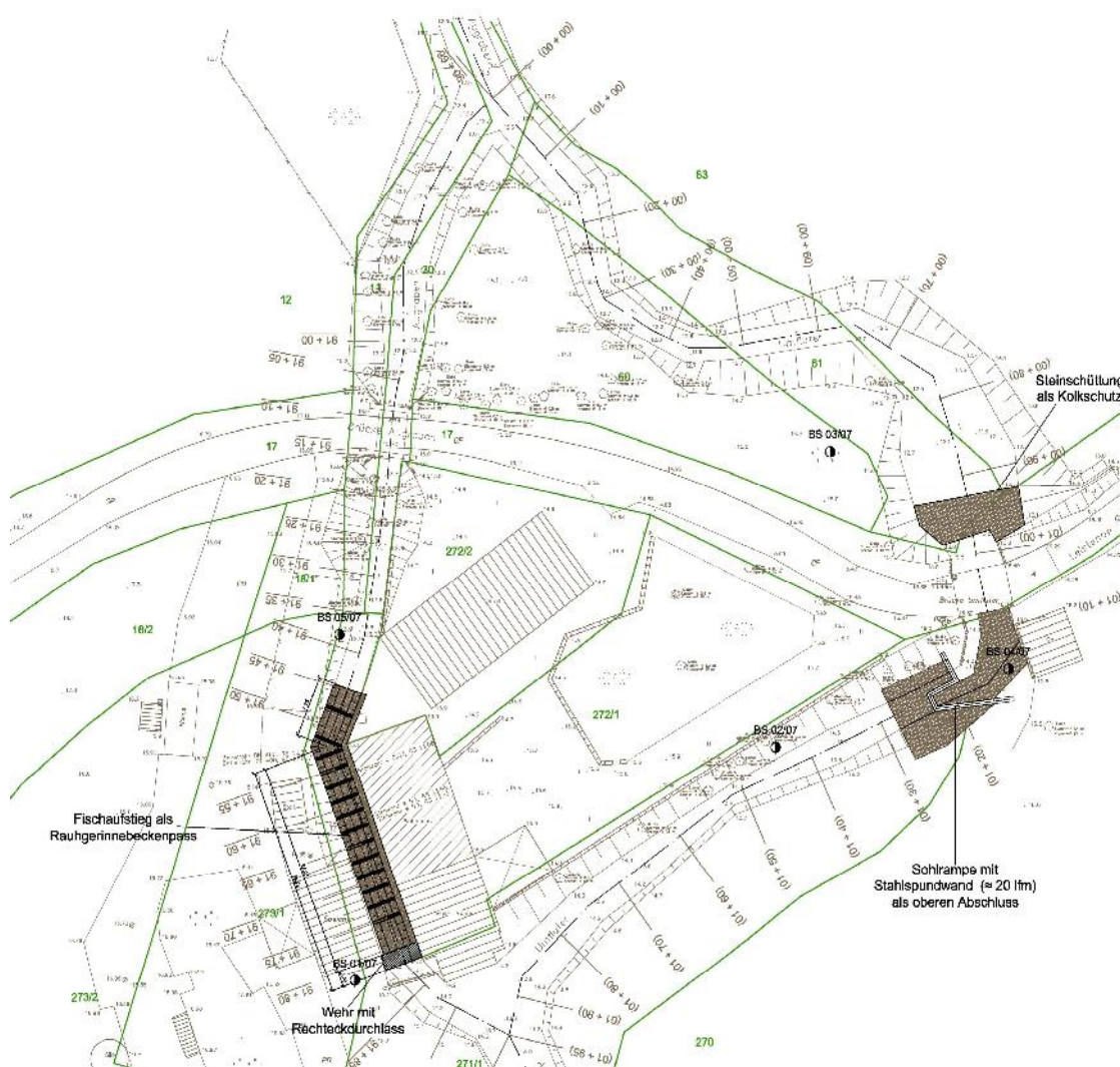
Fischaufstiegsanlage Leistenower Mühle, Lageplan
